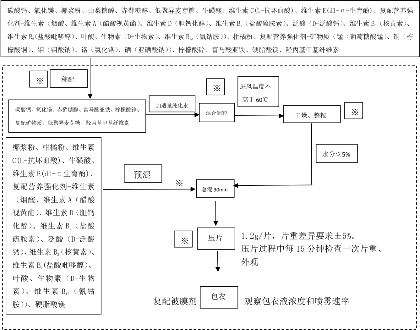
多维多矿片工艺简图
